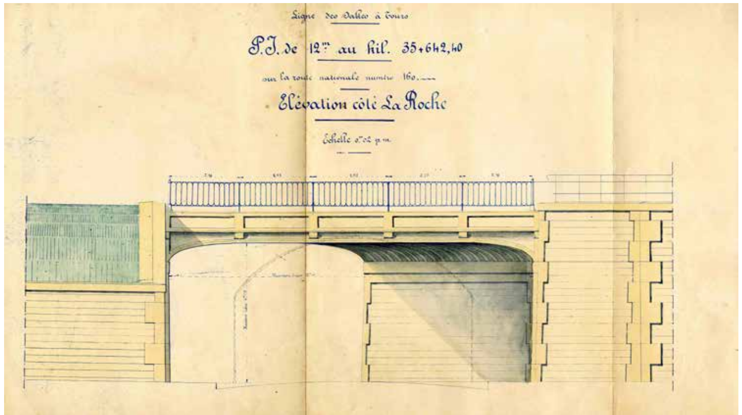
Croquis du Pont Morineau (1926).
